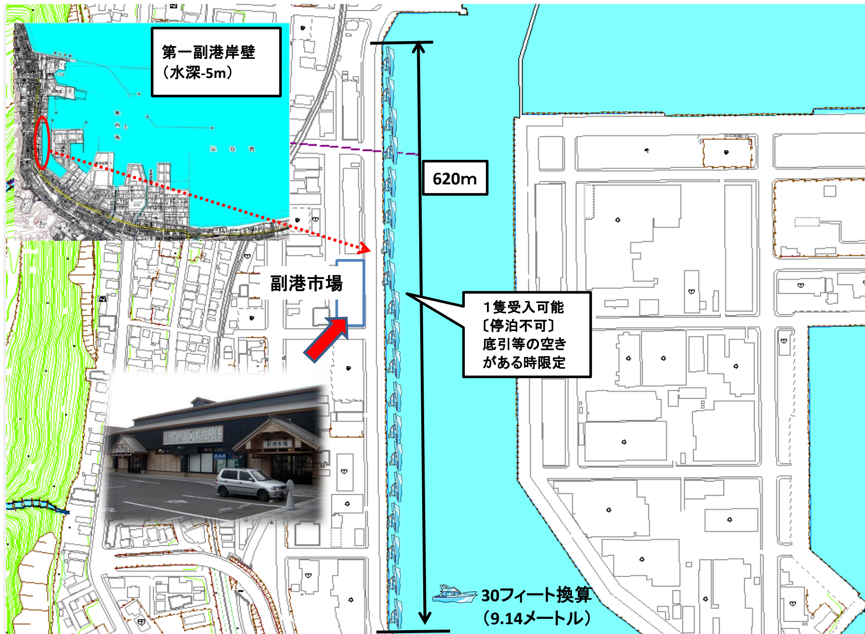
図面【係留岸壁】
