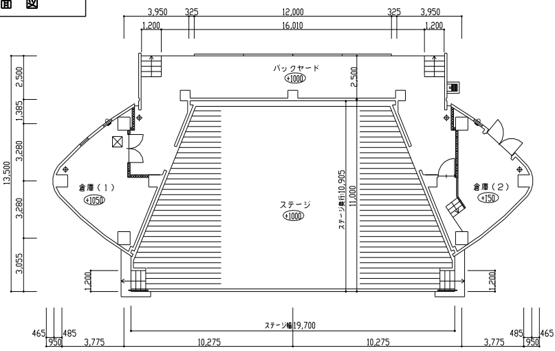
平面図
